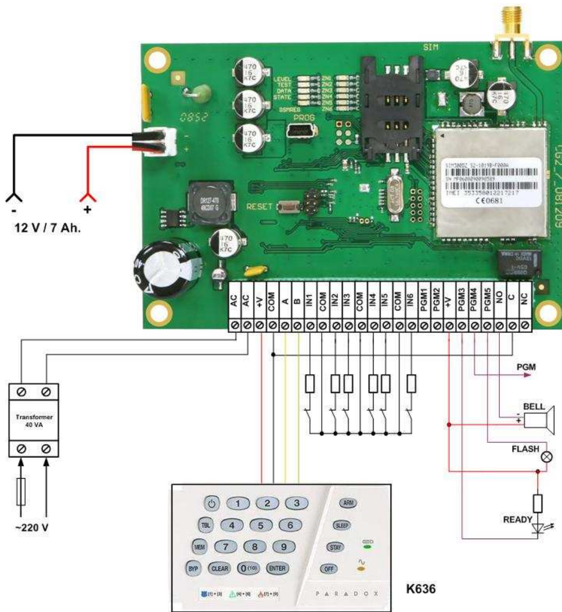
Схема соединений панели CG2 с использованием клавиатуры K636 Paradox®
